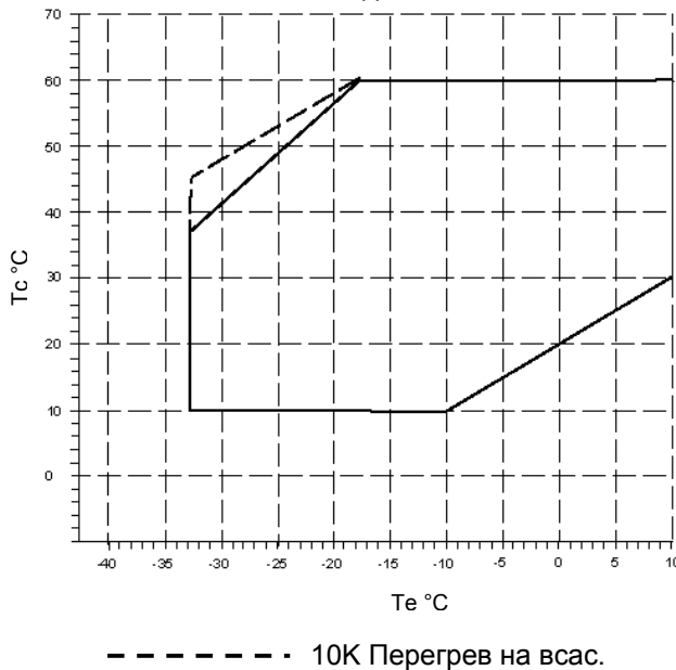
ZB56KCE до ZB11MCE
