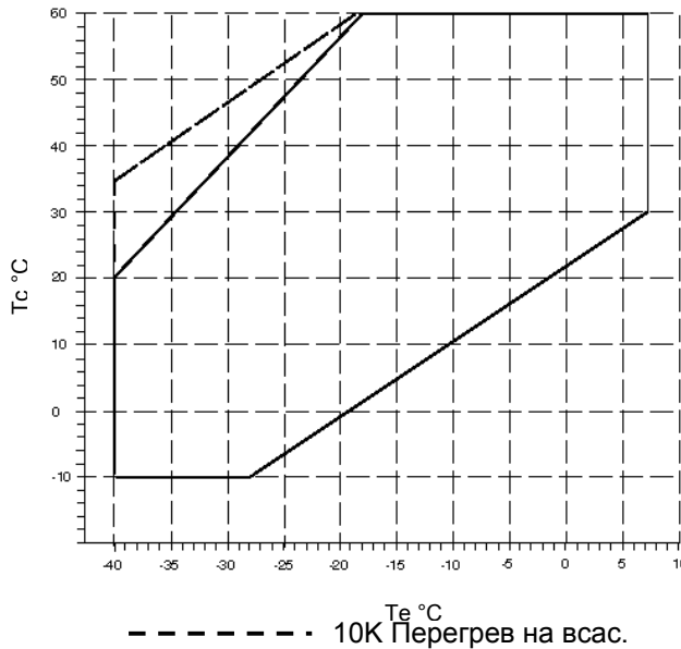
ZS56 до ZS11M3E
