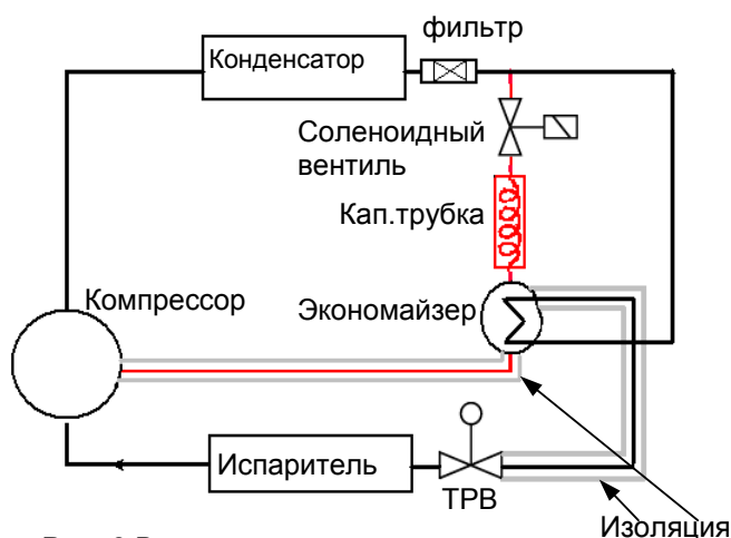
Рис.3 Впрыск пара
