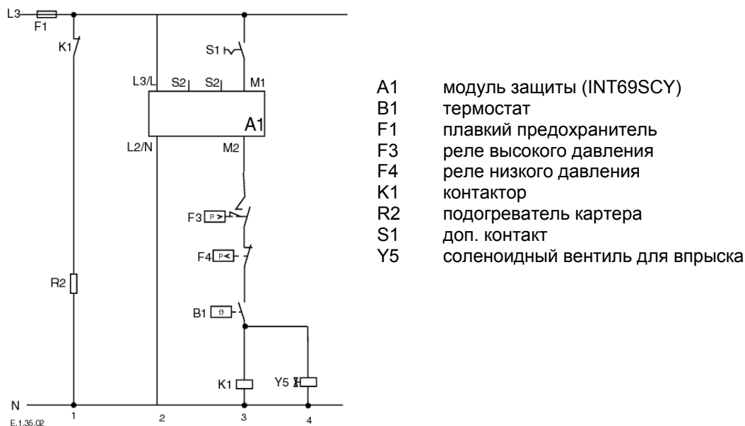
рис. 11: цепь управления компрессором
