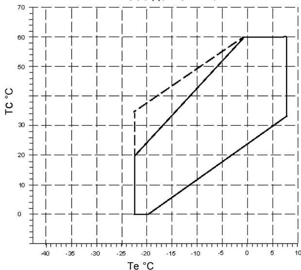
ZS56 до ZS11M3E
